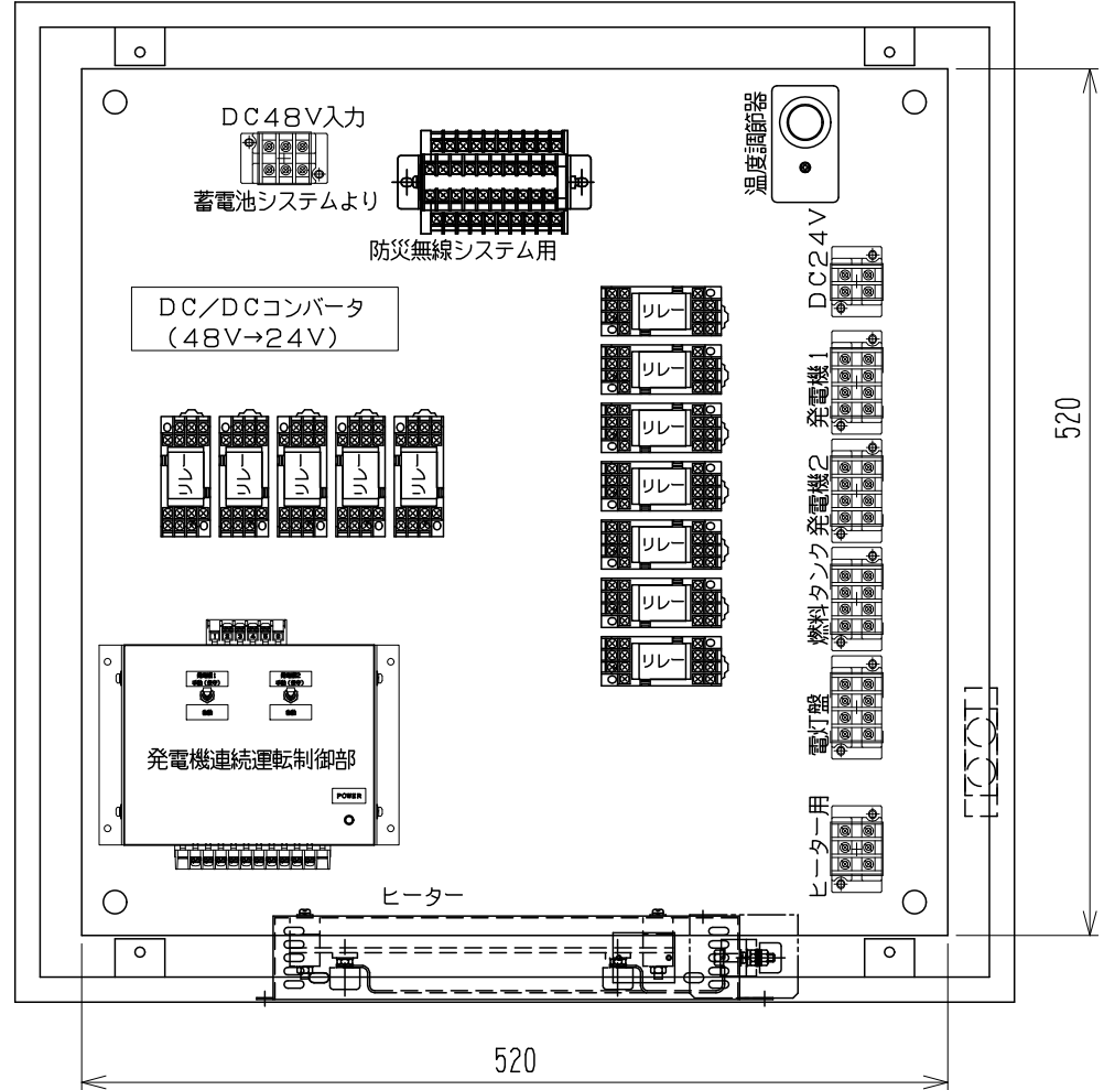
盤内機器配置図
