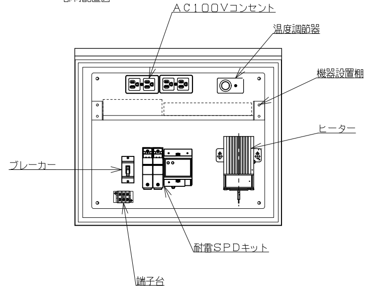
部材配置図
