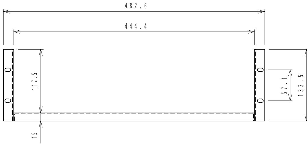
正面図
