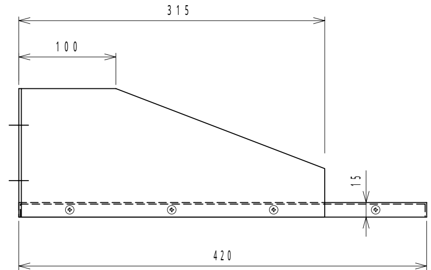
側面図
