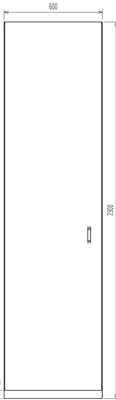
正面図
