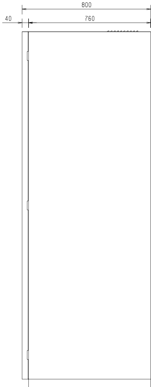
側面図
