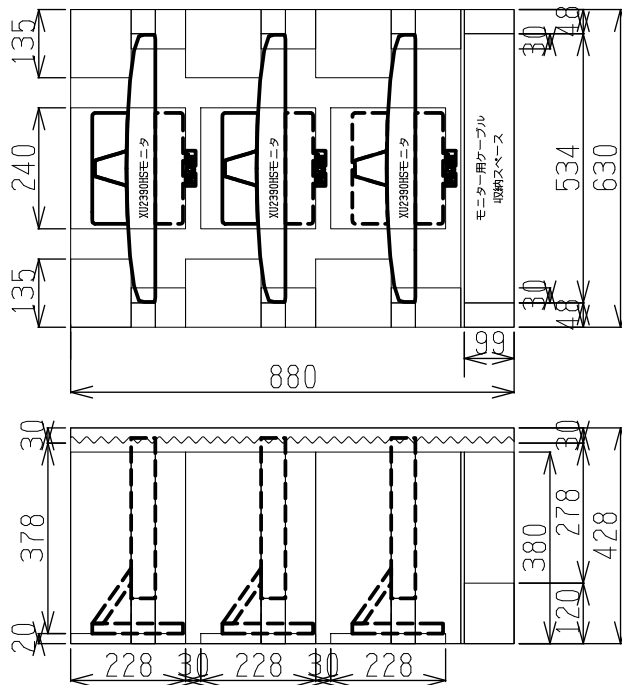
内部図（機器配置図）
