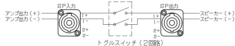
内部回路ブロック
