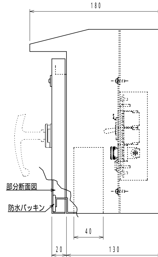
側面図
