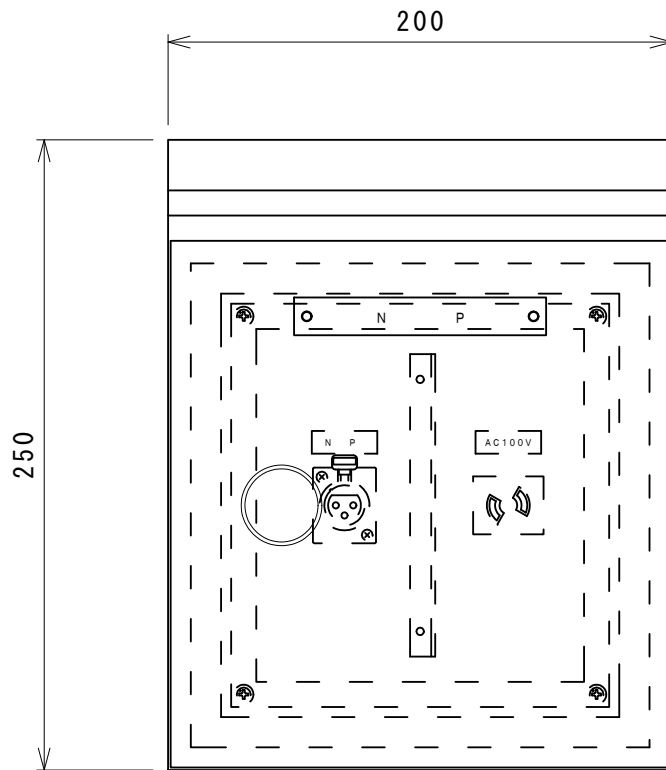
正面図
