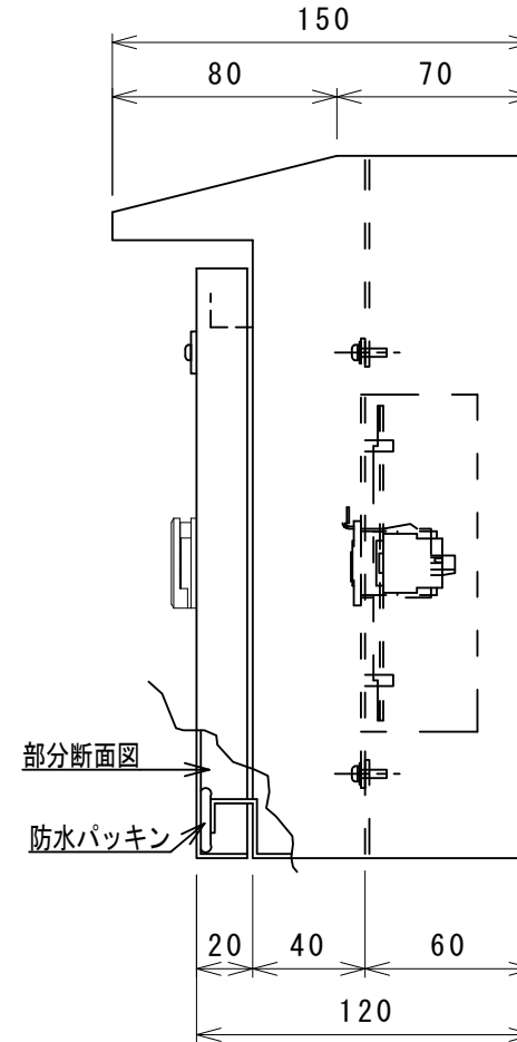
側面図
