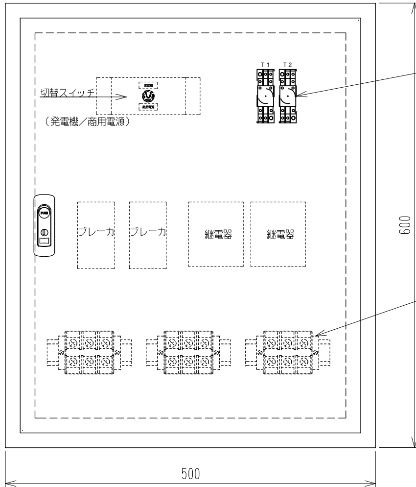
正面図
