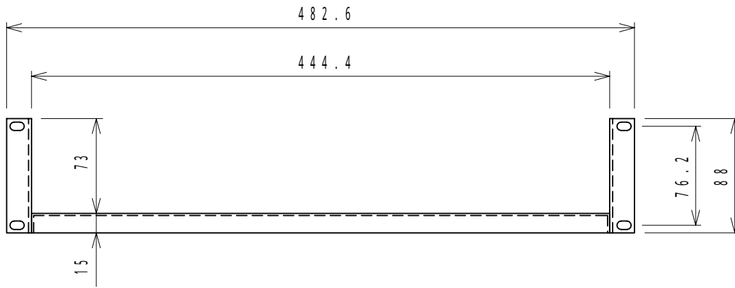
正面図
