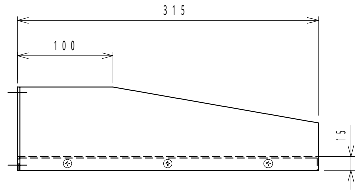
側面図
