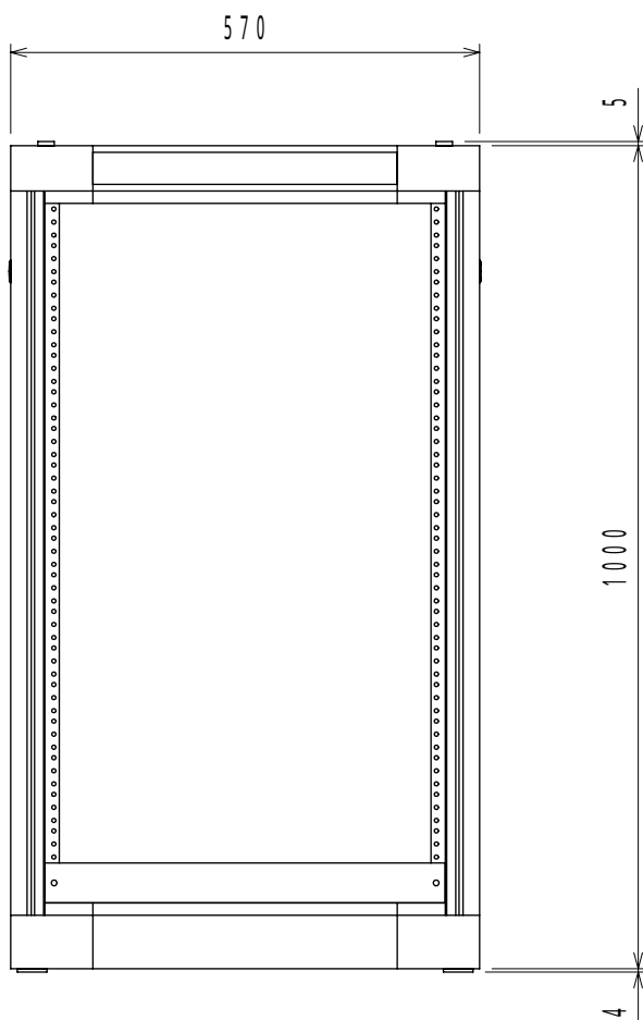
正面図
