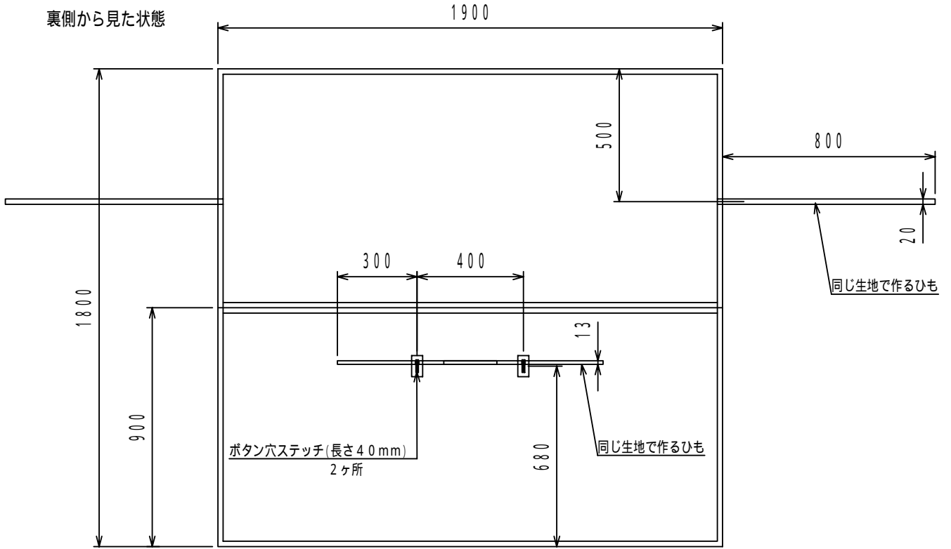
取付例
