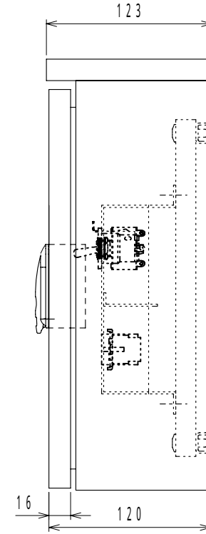
側面図
