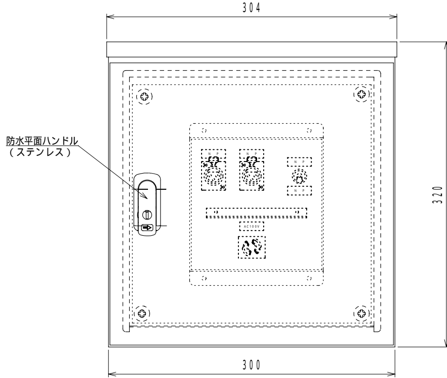
正面図
